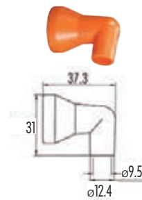
Buse coudée à 90° Ø12.7 mm
