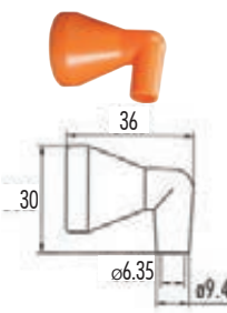
Buse coudée à 90° Ø9.5 mm
