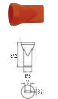
Buse plate L 30 mm à jet concentré
