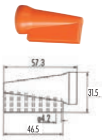
Kit de 4 buses coudées à 90°
