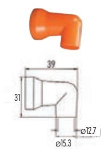
Buse coudée à 90° Ø12.7 mm
